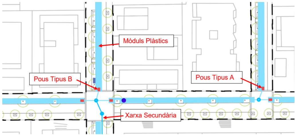
Il·lustració 5. Esquema dels elements de la xarxa de SUDS (Font: Elaboració pròpia)
