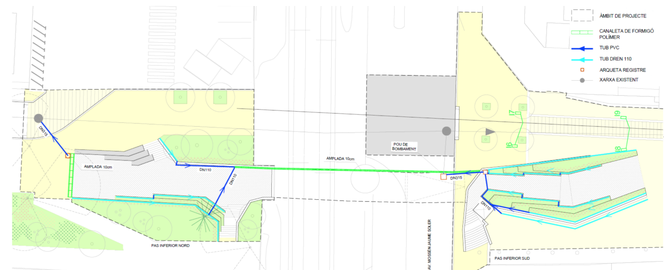
Il·lustració 7. Planta drenatge pas inferior al carrer Sant Pere. (Font: Elaboració pròpia)
