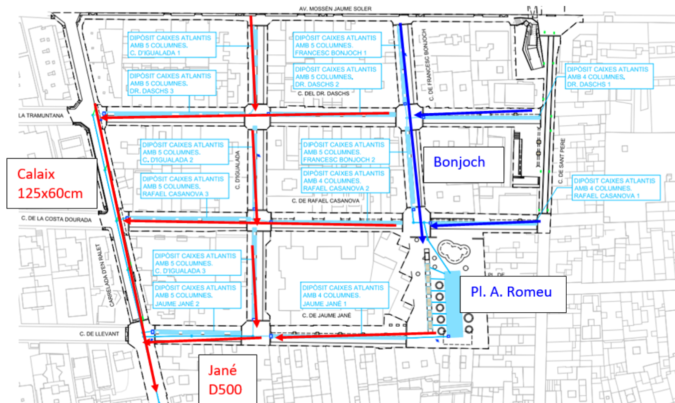
Il·lustració 6. Configuració de dipòsits de caixes segons eixos. En vermell aportacions a l'eix Ralet en blau al dipòsit de la Plaça Alcalde Romeu (Font: Elaboració pròpia).
