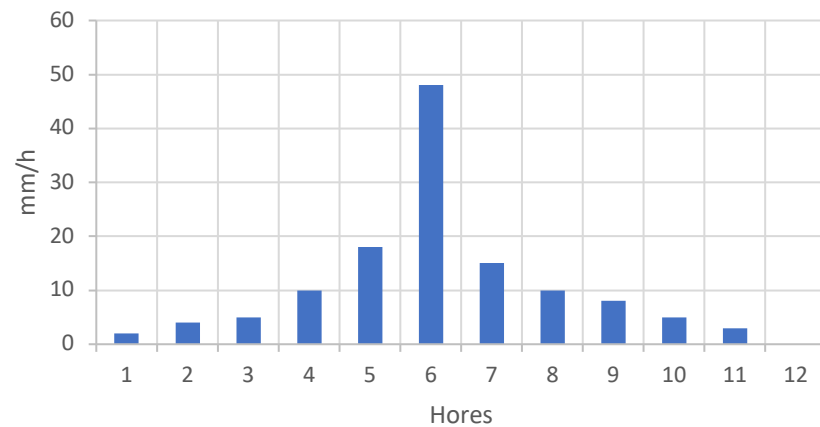
Il·lustració 2. Hietograma de disseny (Font: Pla Director de Clavegueram i Pluvials de Calafell 2010, AGBAR)
