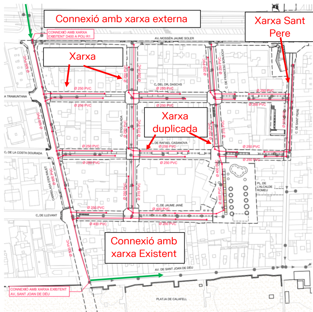
Il·lustració 8. Xarxa de residuals dissenyada de Calafell Platja (Font: Elaboració pròpia)
